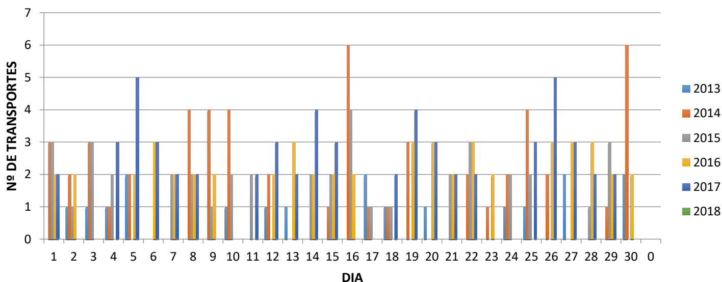
Gráfico 18 - Número de Veículos <3500kg, por dia útil de trabalho – setembro de 2013 a 2018
