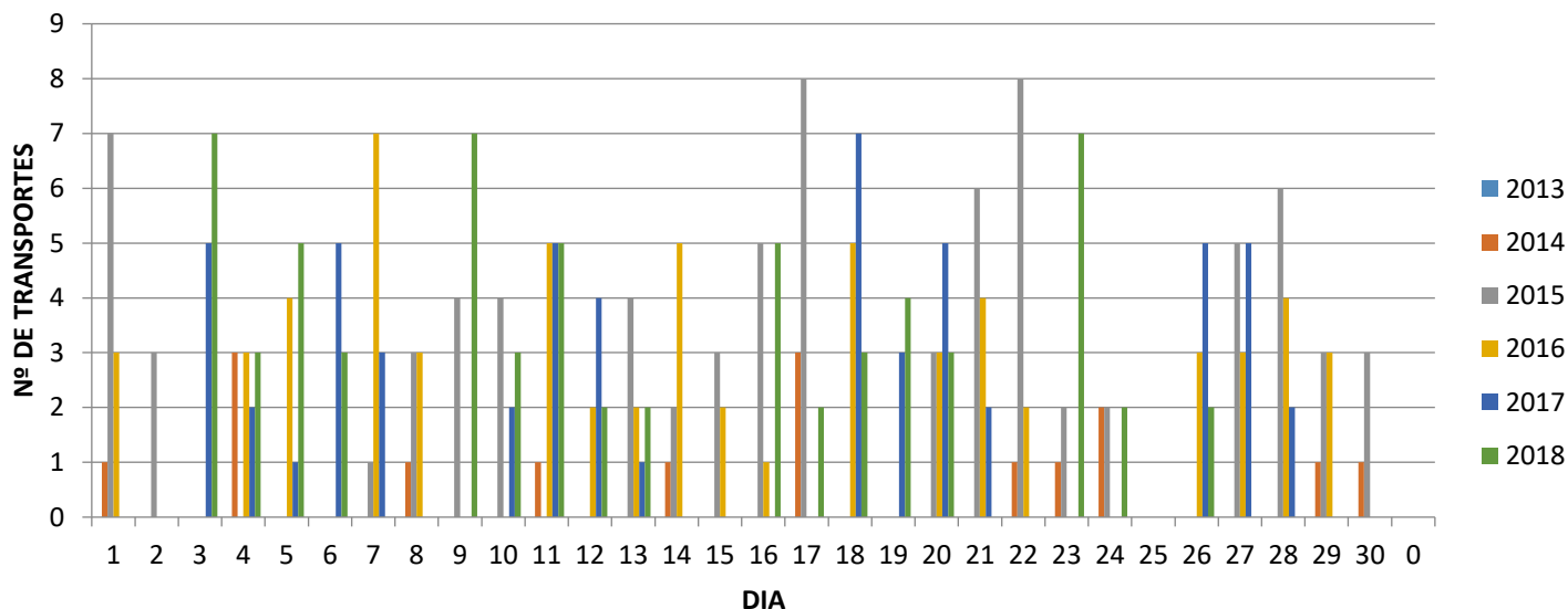
Gráfico 7 - Número de Veículos >3500kg, por dia útil de trabalho – abril de 2013 a 2018
