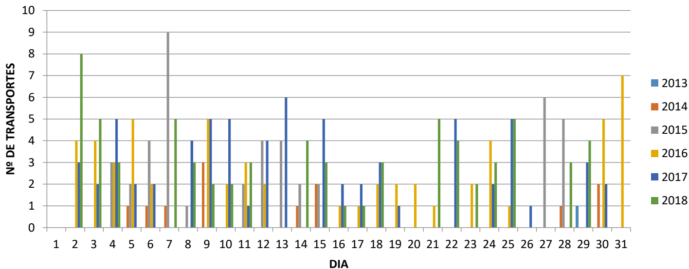
Gráfico 9 - Número de Veículos >3500kg, por dia útil de trabalho – maio de 2013 a 2018
