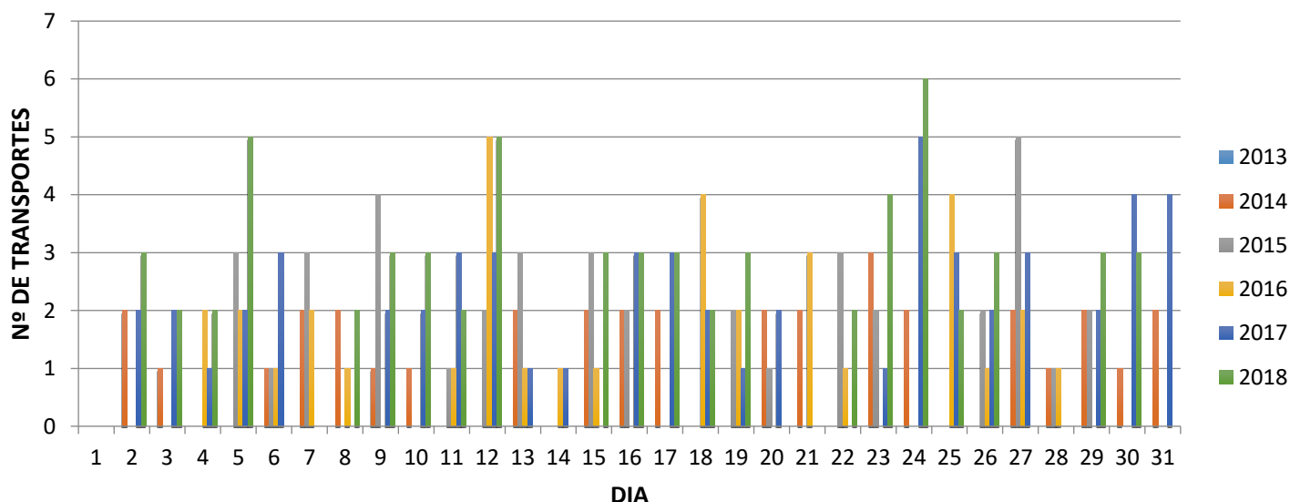
Gráfico 2 - Número de Veículos <3500kg, por dia útil de trabalho – janeiro de 2013 a 2018
