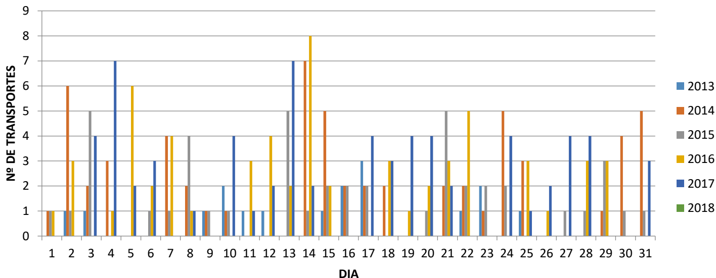
Gráfico 13 - Número de Veículos >3500kg, por dia útil de trabalho – julho de 2013 a 2018
