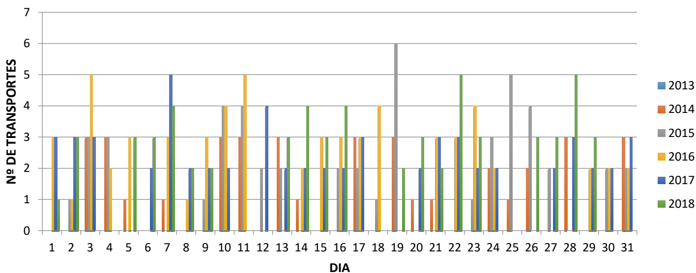
Gráfico 6 - Número de Veículos <3500kg, por dia útil de trabalho – março de 2013 a 2018
