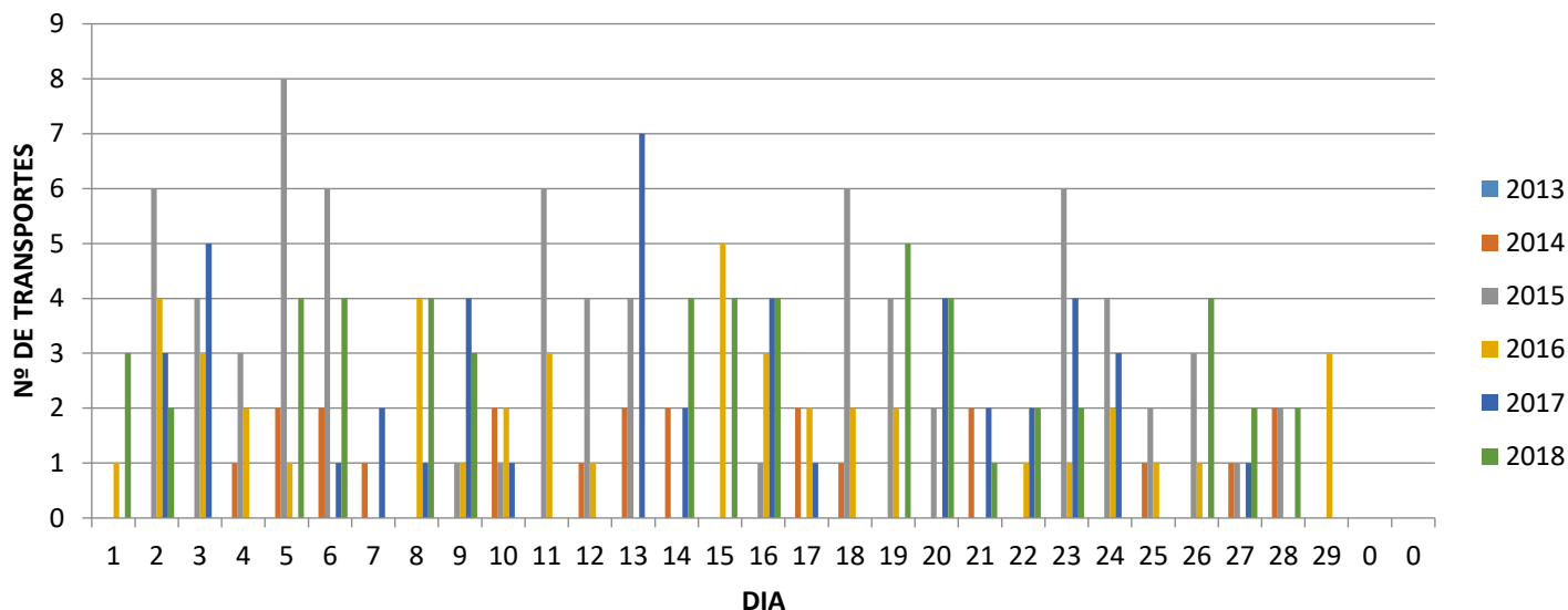
Gráfico 3 - Número de Veículos >3500kg, por dia útil de trabalho – fevereiro de 2013 a 2018
